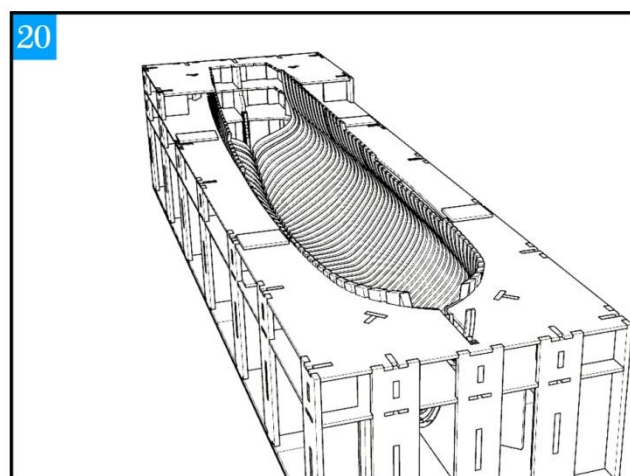
安顺序安装肋骨
