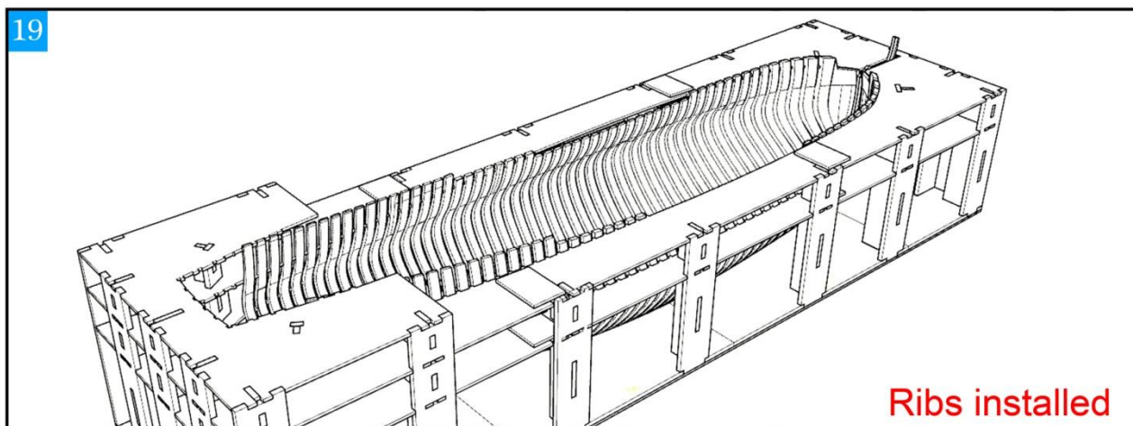
安顺序安装肋骨
