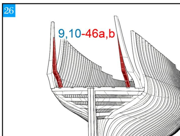
顶部斜向打磨后安装
