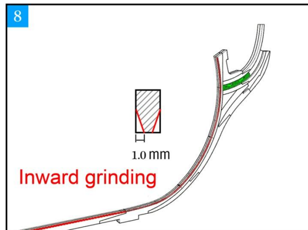
按打磨线打磨 向内1.0mm
