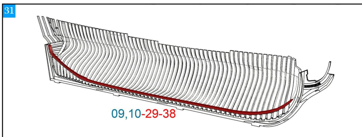
安装内龙骨
