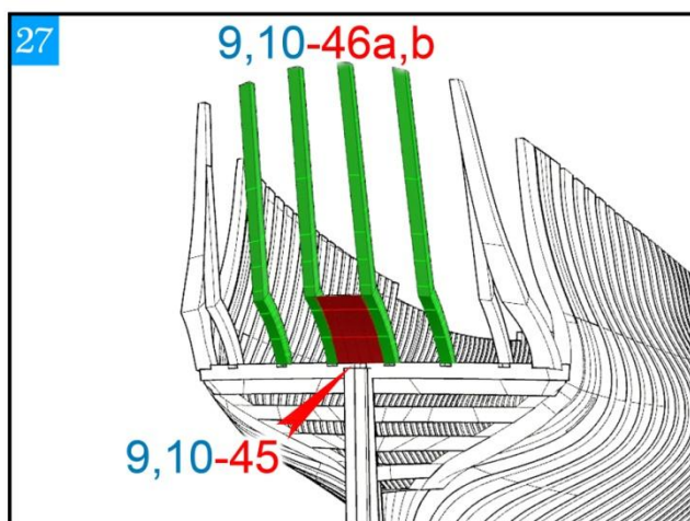
制作尾部
