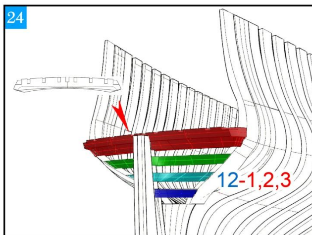
安装尾部
