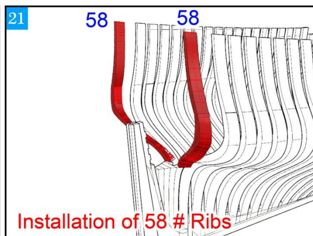
制作58#弯肋骨
