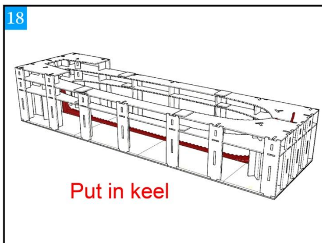
放置龙骨
